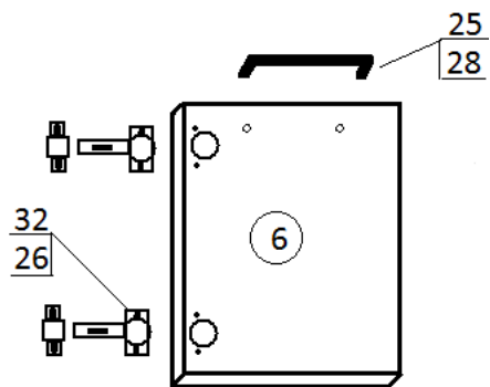
Рис. 1. Схема сборки фасада
