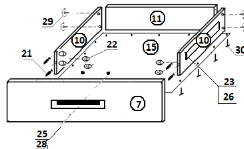
Рис.3. Схема сборки ящика
