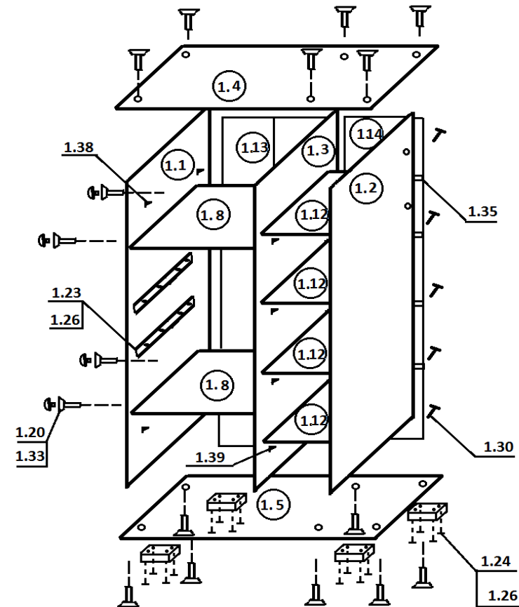
Рис.3. Схема сборки ящика
