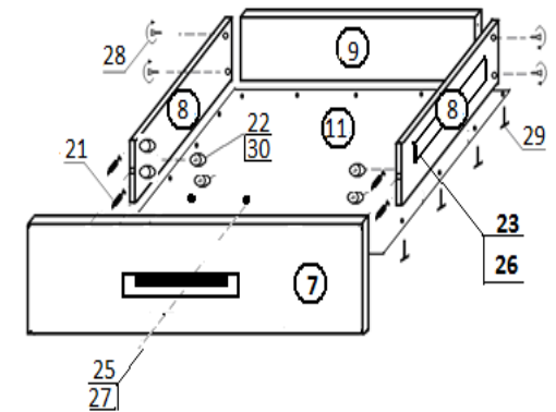
Рис. 3. Сборка ящика
