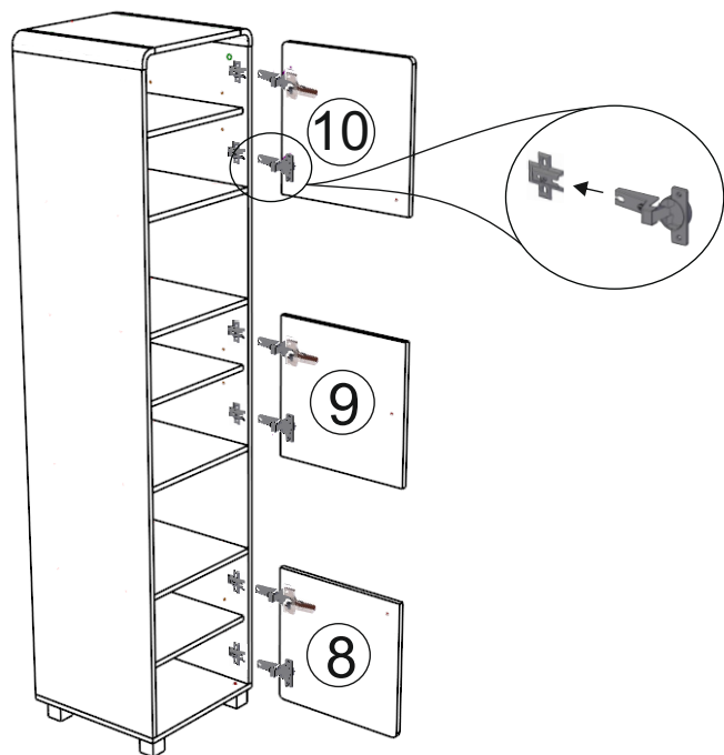
Рис.5. Установите фасады
