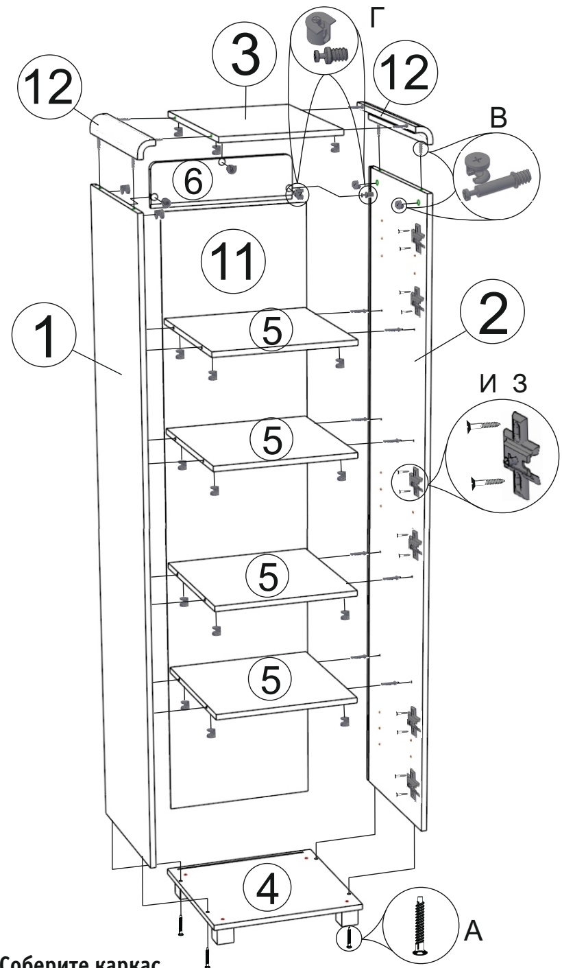
Рис. 3. Соберите каркас
