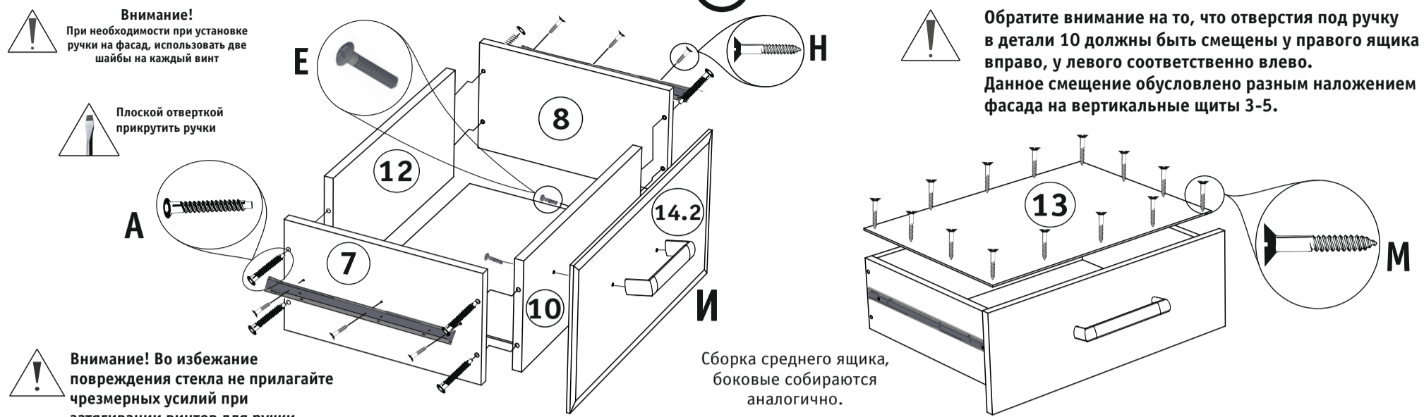
Рис. 1. Сборка ящика.
