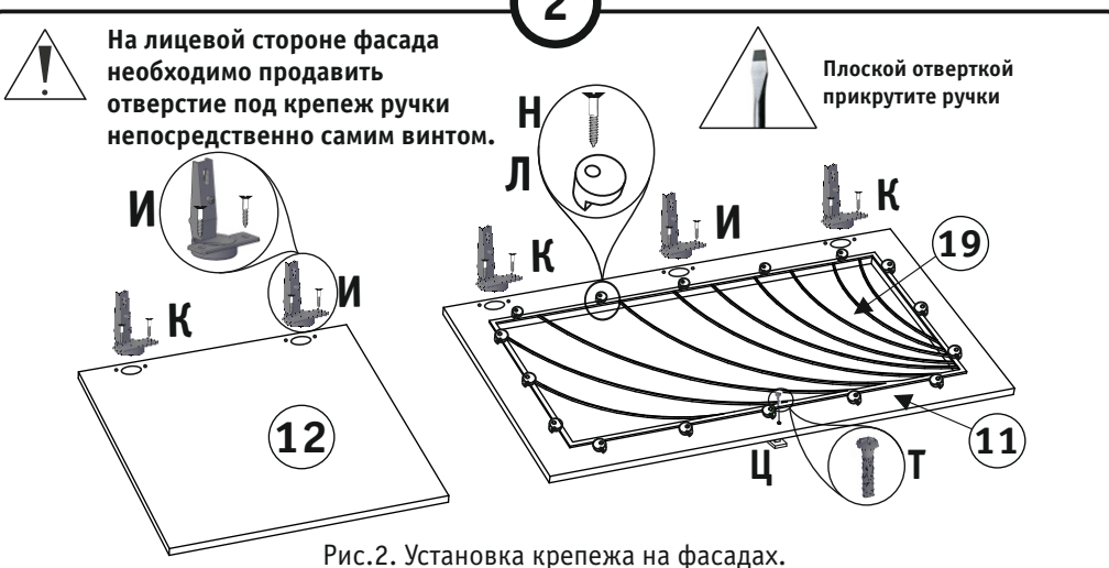
Рис.2. Установка крепежа на фасадах.
