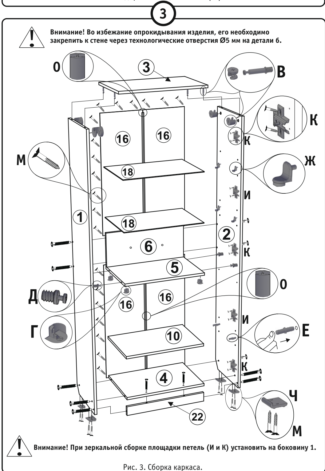
Рис. 3. Сборка каркаса.
