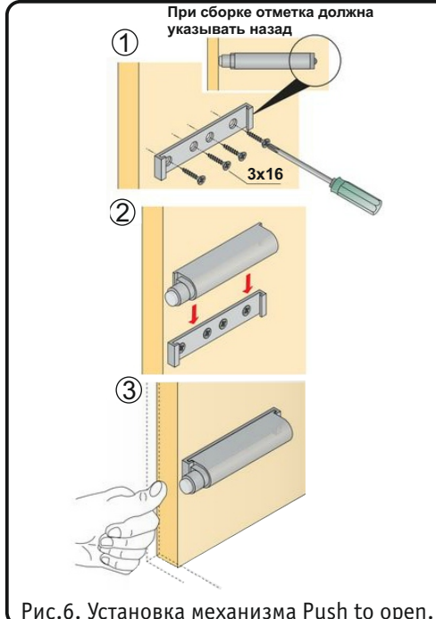
Рис.6. Установка механизма Push to open.
