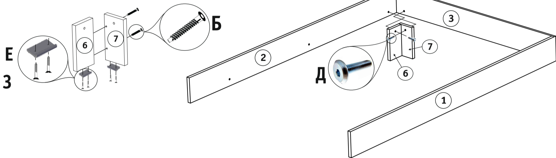
Рис. 2. Установка опор.
