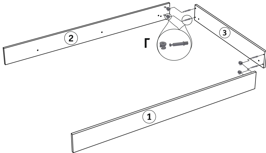
Рис. 1. Сборка основания.
