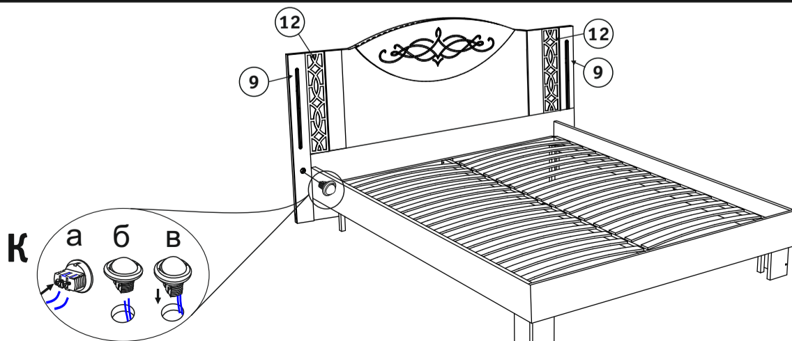
Рис. 4. Установка выключателя.
