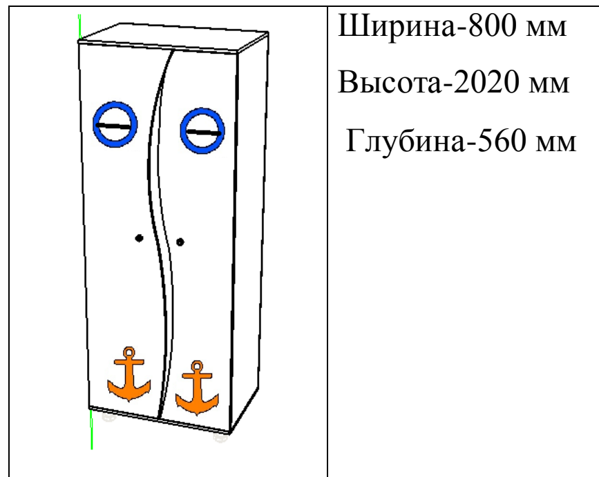
Рис.1. Общий вид шкафа.
